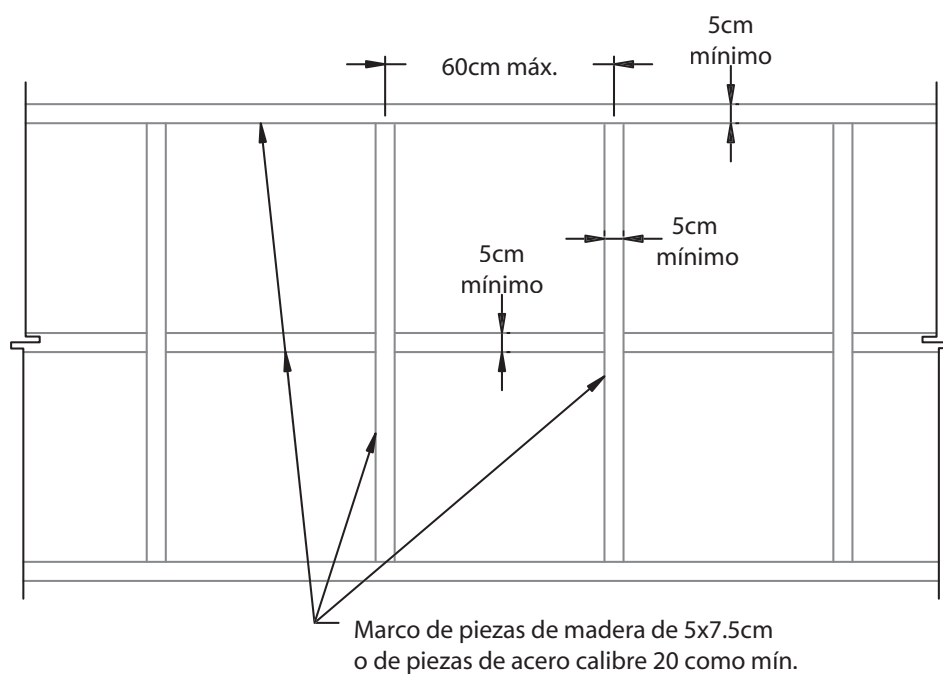
Fig. 17.17. Paredes delgadas a doble forro.
