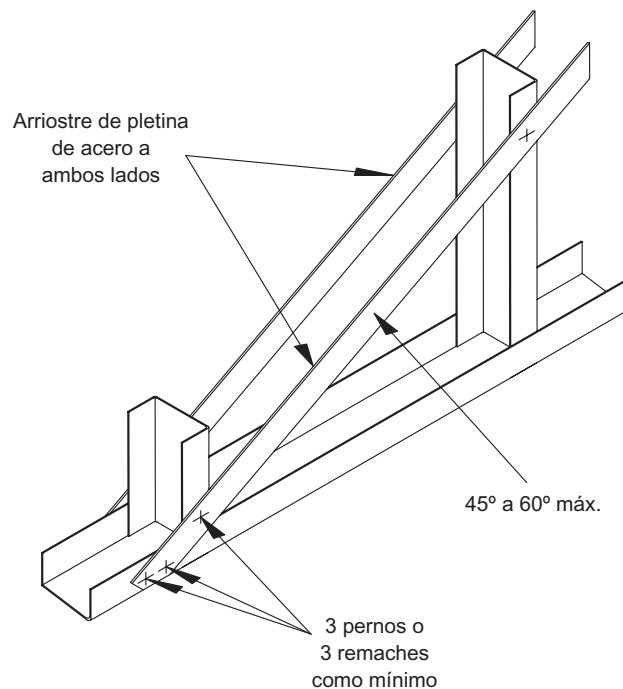
Fig. 17.19. Arriostre de paredes a doble forro.
