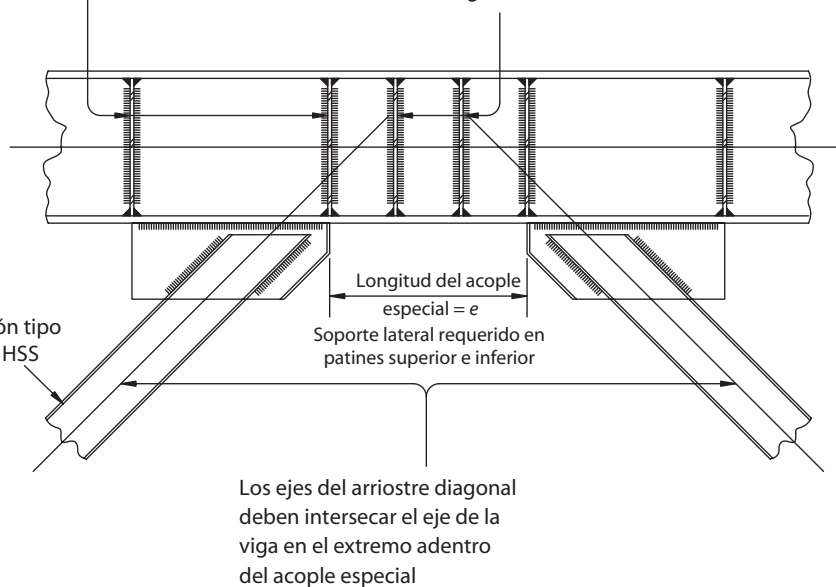
Figura 10.5. Detalles de acoples especiales , Ref.7.
