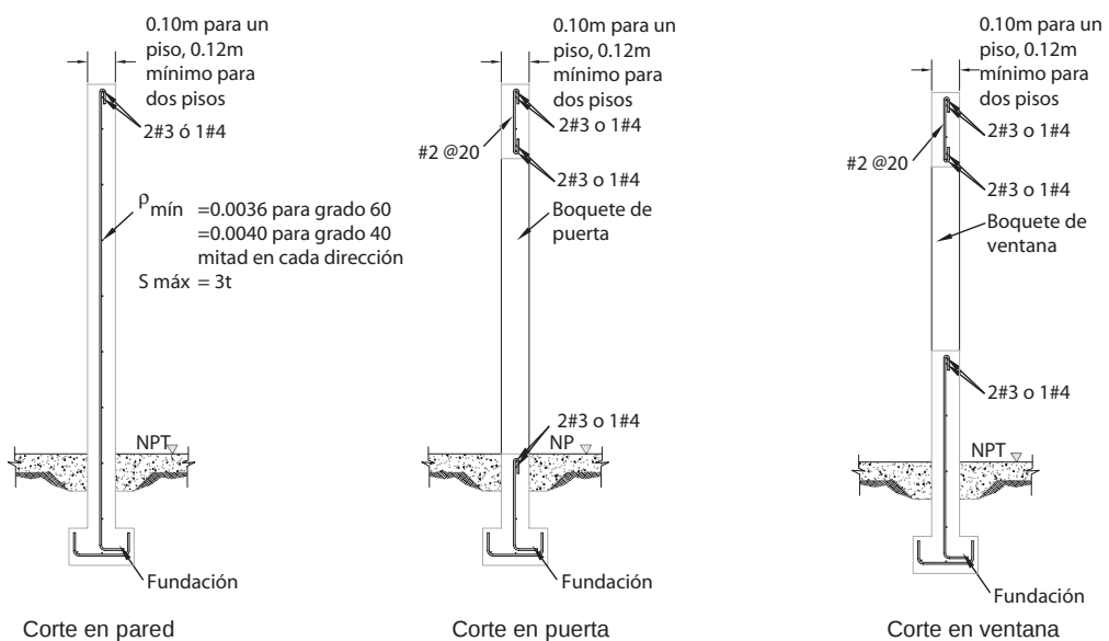
Fig. 17.14. Cortes en paredes de concreto reforzado.
