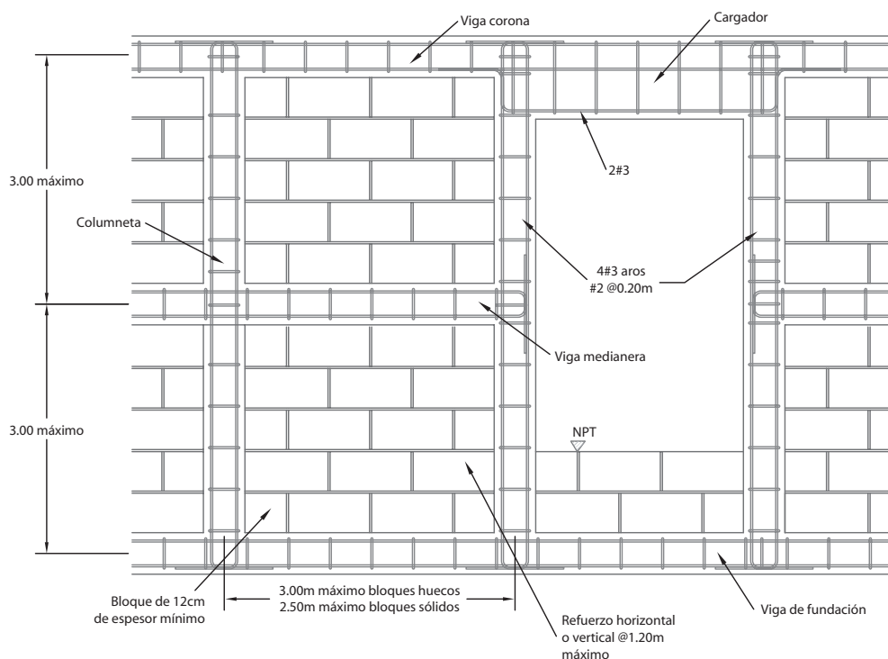
Fig. 17.11. Elevación de un marco relleno de mampostería.
